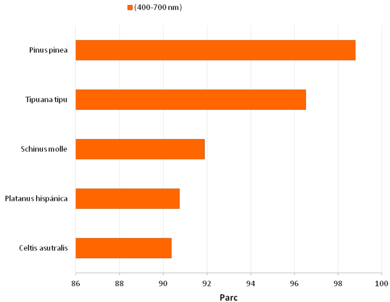
Figura 1. Valores de atenuación (%) de la radiación solar de entrada (400-700 nm) de las especies presentes en el Parc de Alhambra.
